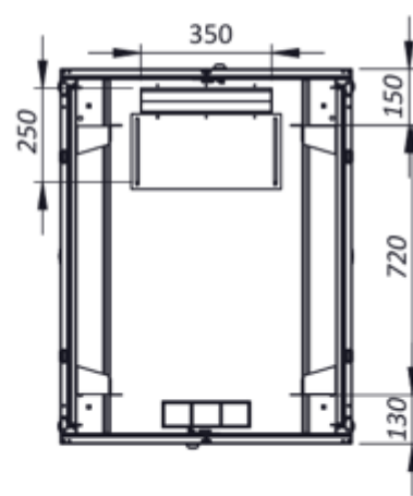
Vue détaillée
